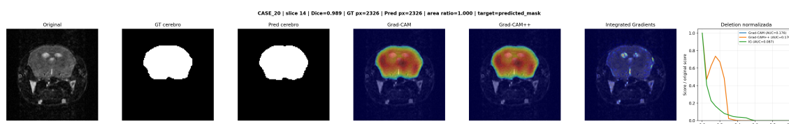
Figura 3.10: Ejemplo de visualización generada por el procedimiento de explicabilidad aplicado al modelo de segmentación cerebral. Se muestran, de izquierda a derecha, el corte original de RMN, la máscara de referencia, la máscara predicha por el modelo y los mapas de relevancia obtenidos mediante distintos métodos de explicabilidad. Esta figura ilustra el tipo de salida utilizada para el análisis cualitativo del comportamiento del modelo.
