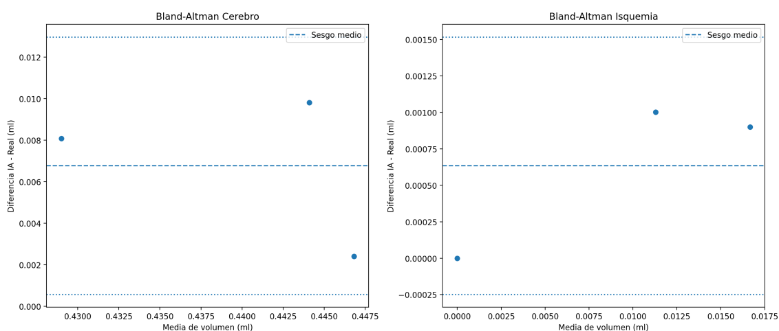
Figura 4.7: bland altman
