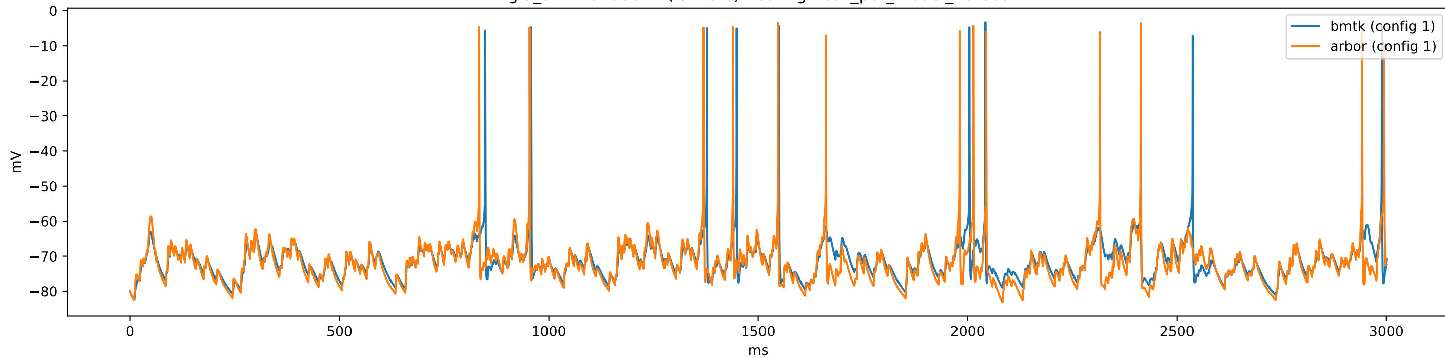
gid_92-478793814 (i5Pvalb) - config.1cell_per_model_iclamp
