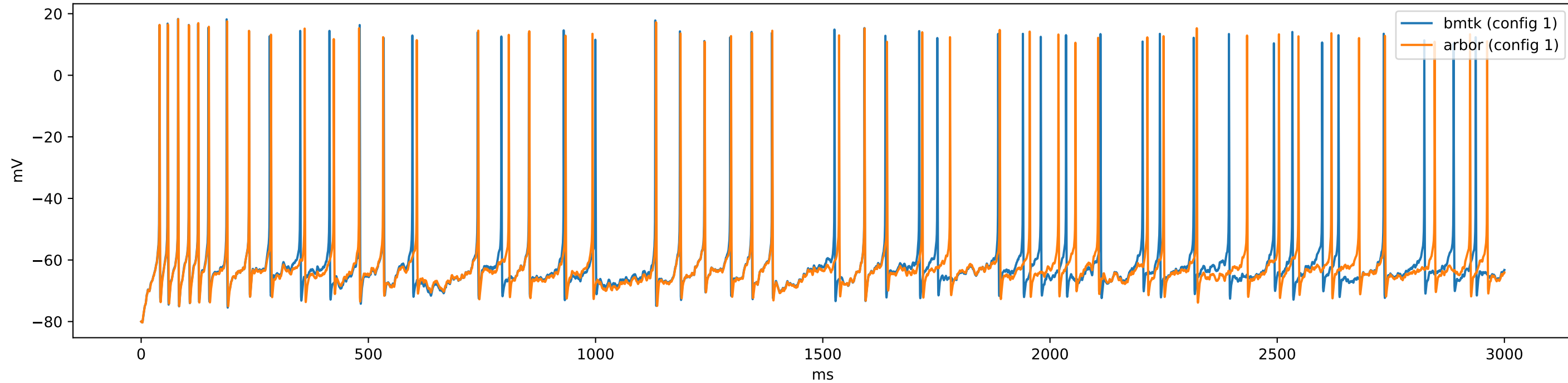
gid_3-327962063 (i23Htr3a) - config.1cell_per_model_iclamp
