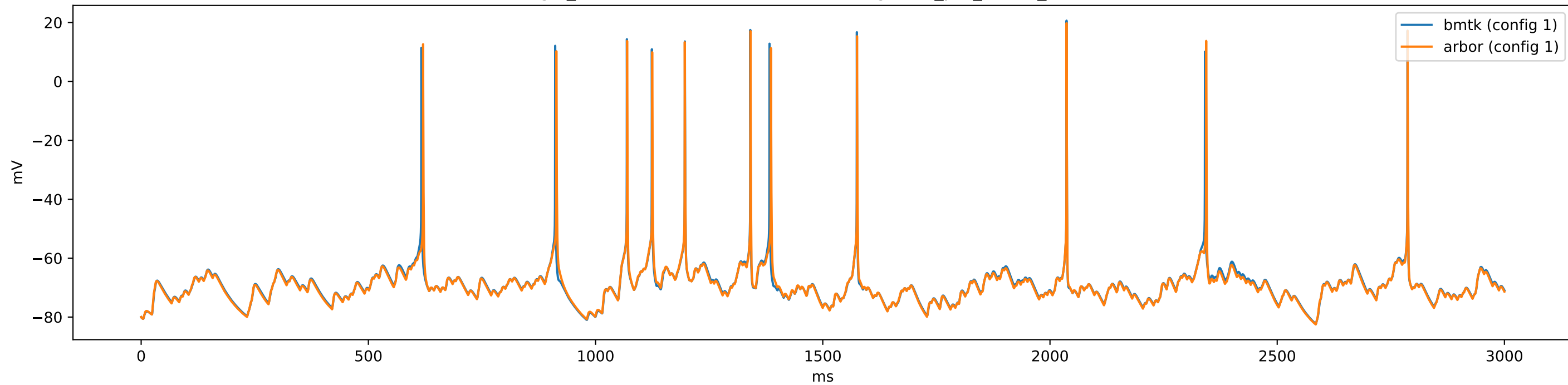
gid_38-314900022 (e4Scnn1a) - config.1cell_per_model_iclamp
