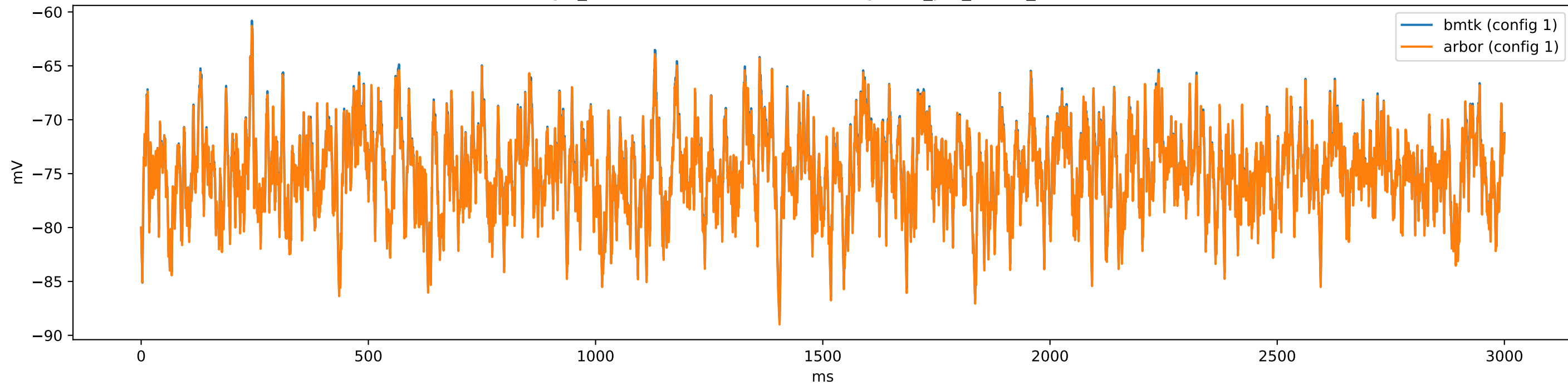
gid_5-469753383 (i23Htr3a) - config.1cell_per_model_iclamp
