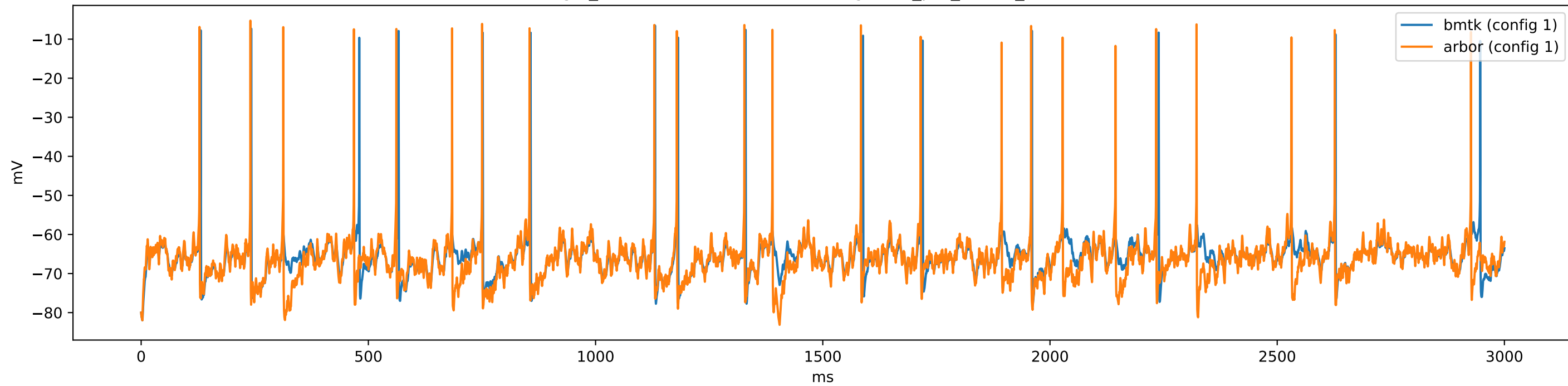
gid_52-313862167 (i4Sst) - config.1cell_per_model_iclamp
