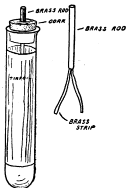
FIG. 224. — A Test-Tube Leyden Jar.
