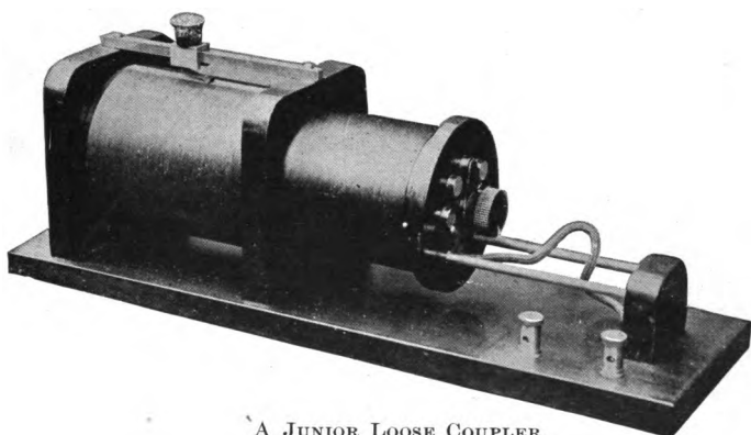
A JUNIOR LOOSE COUPLER.
