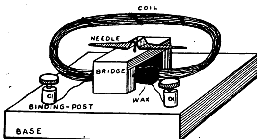
FIG. 111. — Galvanoscope.
