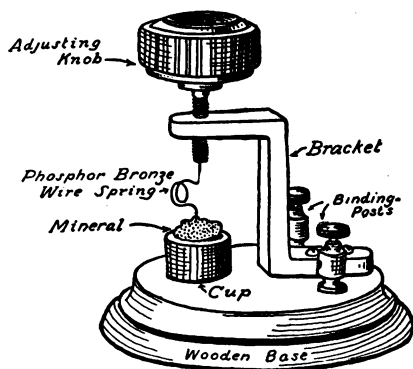
FIG. 210. — A Crystal Detector.
