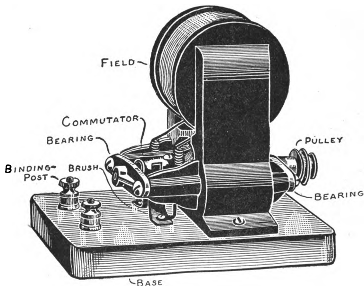
FIG. 262. — Complete Dynamo.
