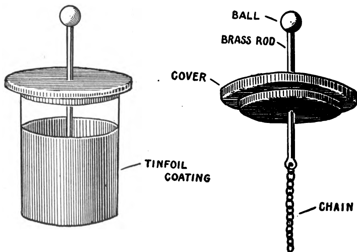
FIG. 45. — The Leyden Jar.
