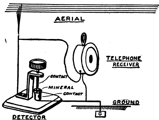
FIG. 195. — A Simple Receptor.
