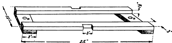
FIG. 37. — The Frame.
