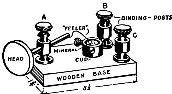
FIG. 214. — "Cat-Whisker" Detector.
