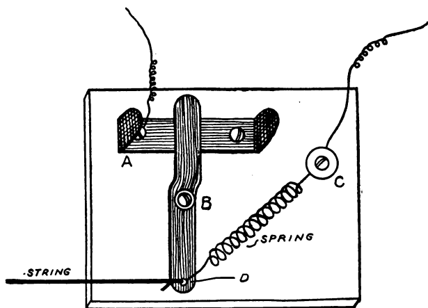
FIG. 125. — Burglar-Alarm Trap.
