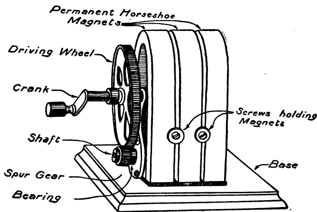
FIG. 251. — A Telephone Magneto.
