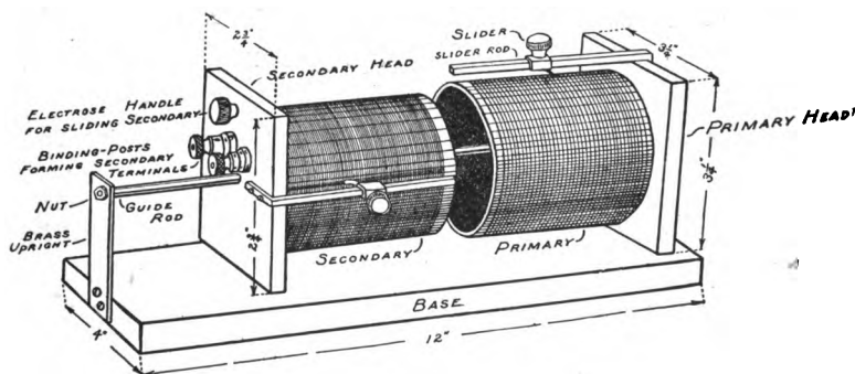
FIG. 204. — A Simple Loose Coupler.
