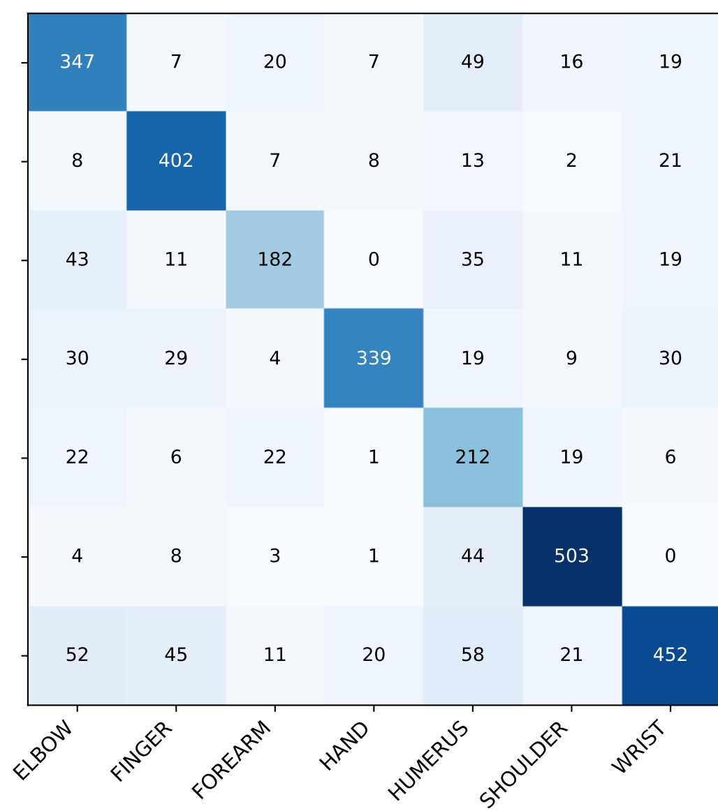
v2 SENet — 64-ref (76.2%)
