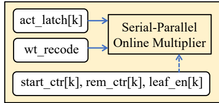
(d) Single Leaf Microarchitecture
