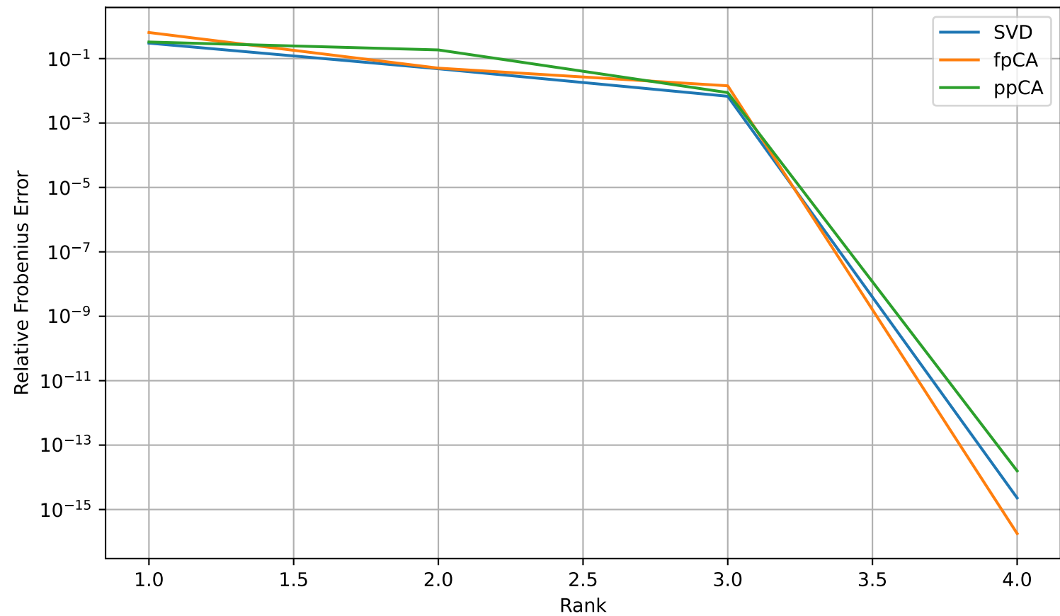
Iris Linear
