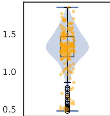
1 m_mode
