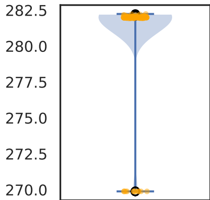
1 L_mode
