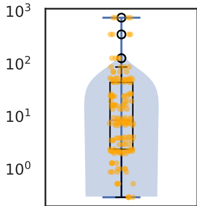
1 e_mode_geommean
