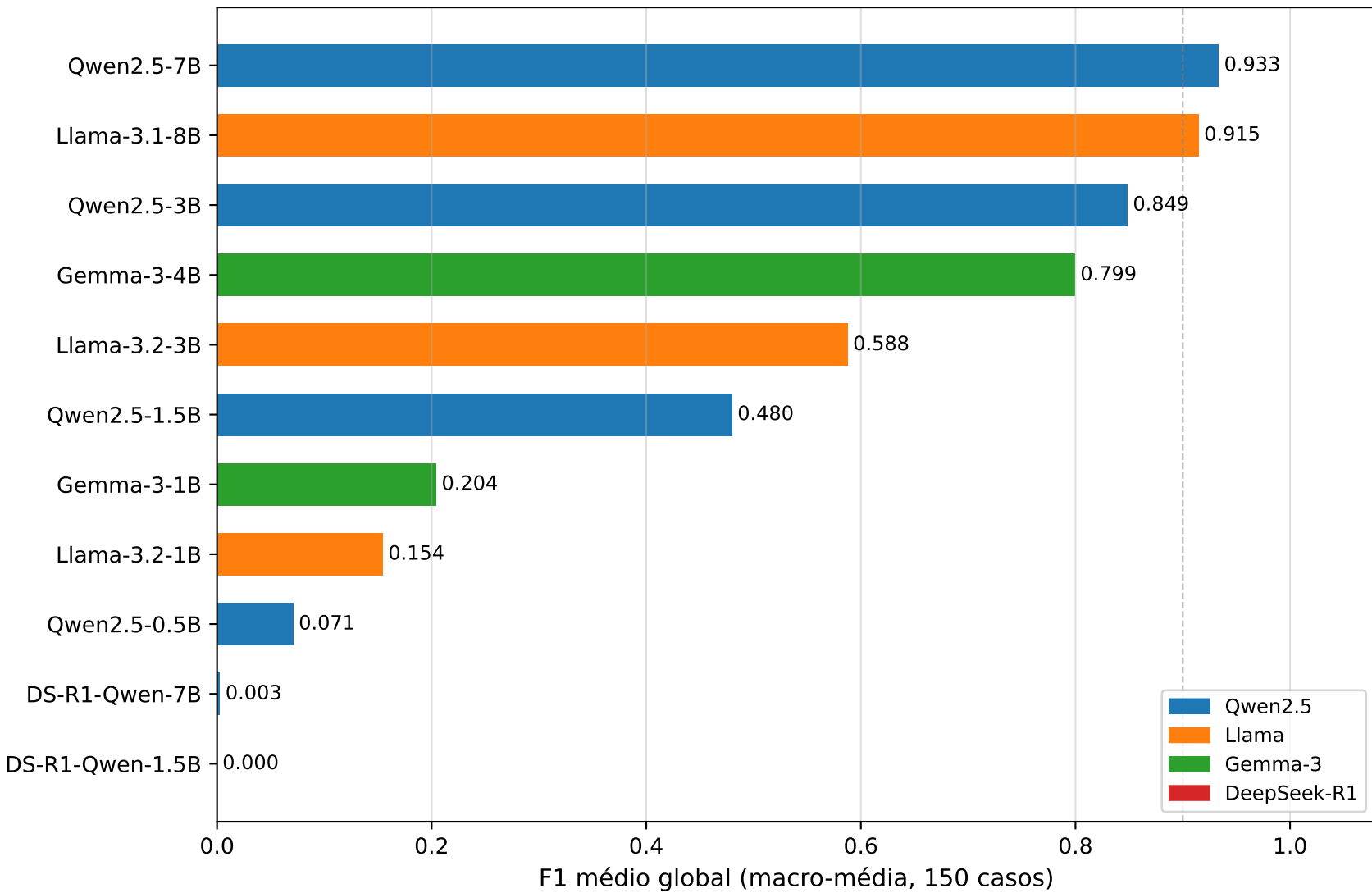
Exp 1 — Efeito da dimensão do modelo (bf16)
