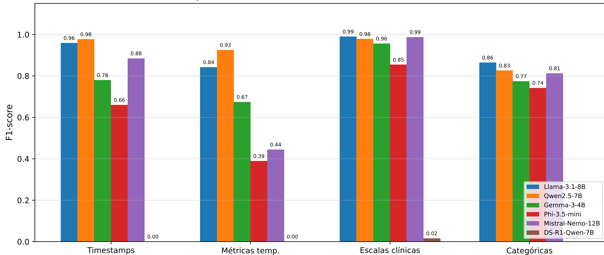
Exp 2 — Efeito da família/receita de treino (~7-12B, bf16)
