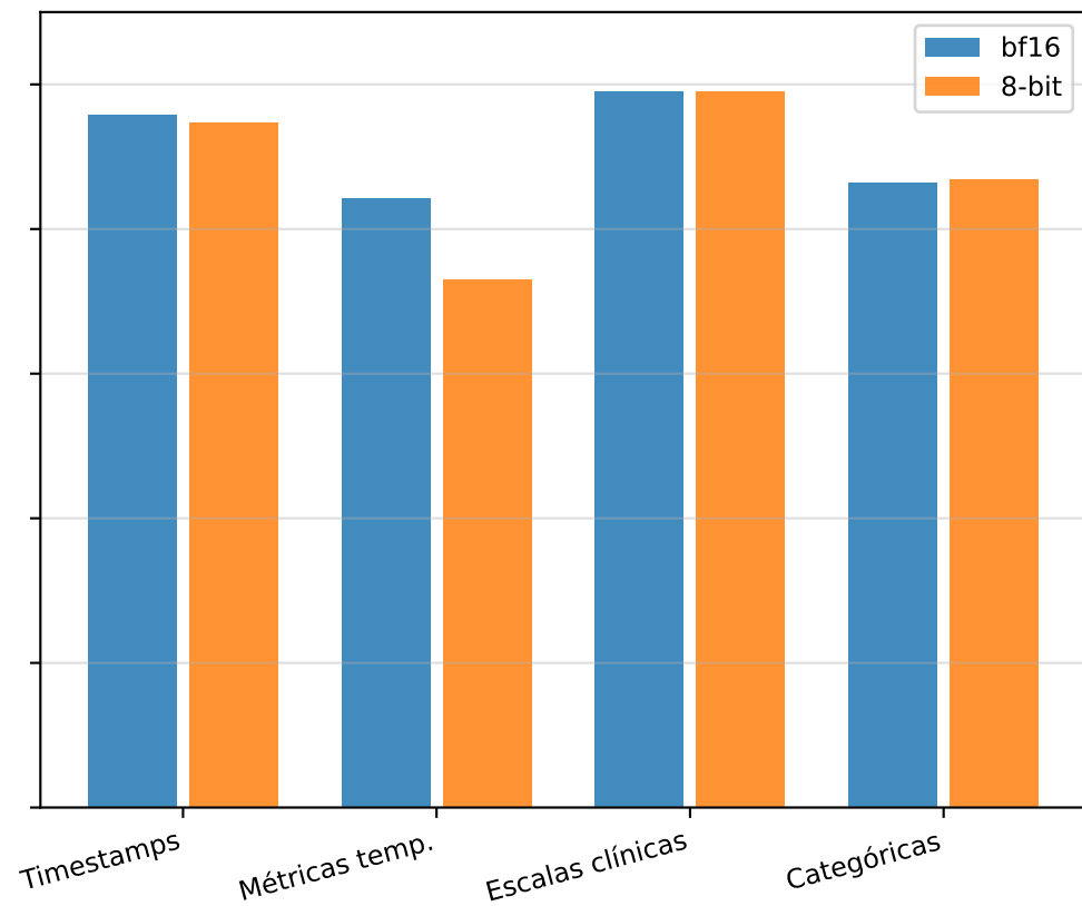
Llama-3.1-8B
