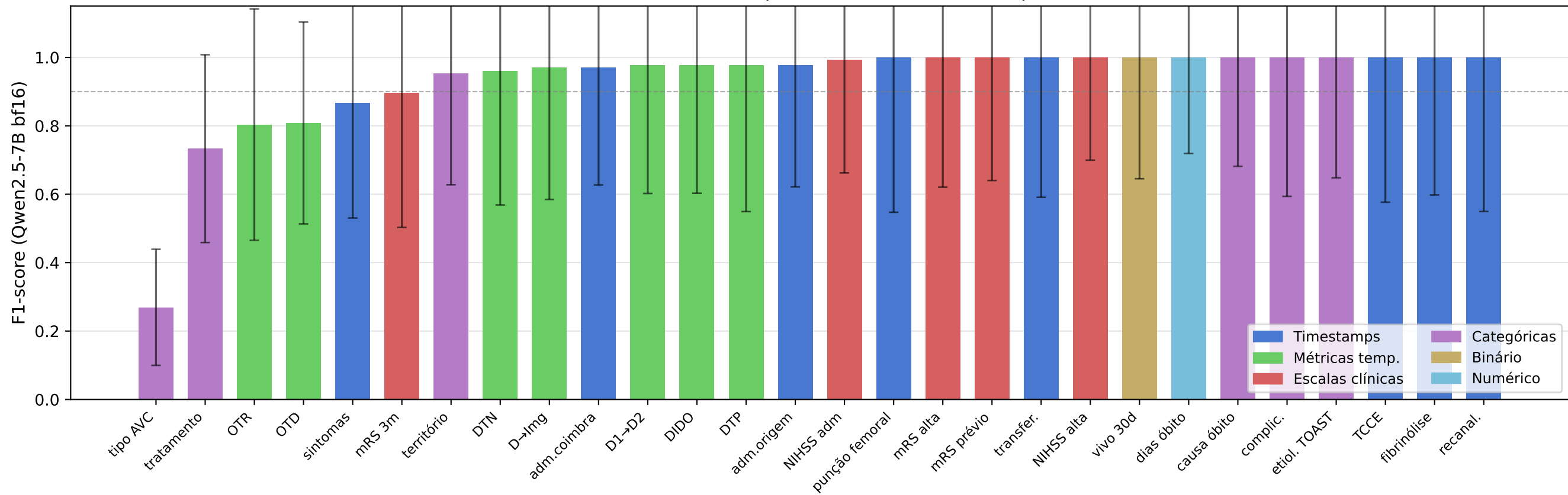
F1-score por variável individual — Qwen2.5-7B (barras de erro = desvio padrão entre modelos competentes)
