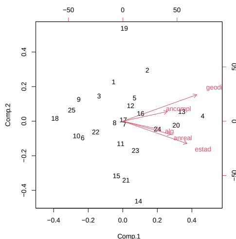
Figura 4.3.: Biplot
