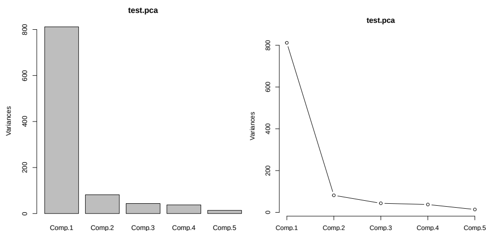
Figura 4.1.: Gráficos de sedimentación.
