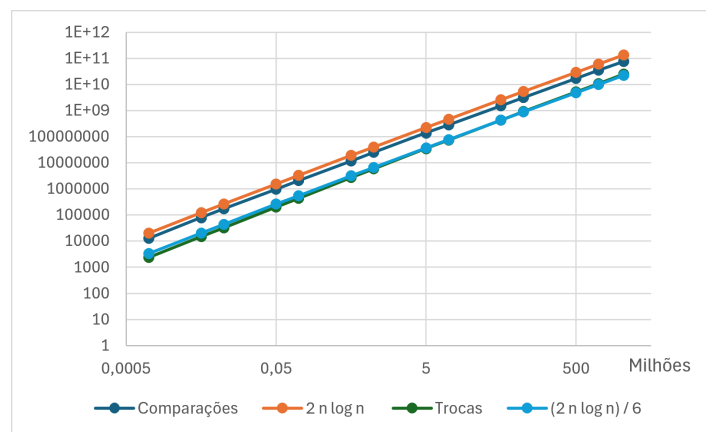
Figura 5: Comparativo entre o número de comparações e trocas e seu comportamento esperado para o melhor caso do quick sort. Escala dilog.
