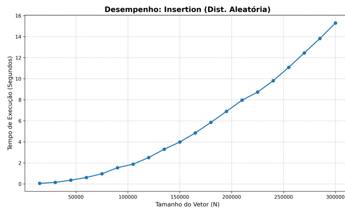
Figura 4: Desempenho Insertion Sort: distribuição aleatória
