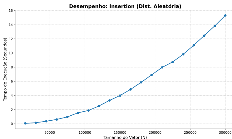
Figura 2: Desempenho Insertion Sort: distribuição aleatória
