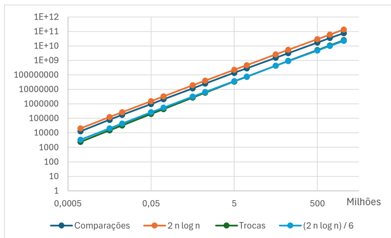
Figura 3: Comparativo entre o número de comparações e trocas e seu comportamento esperado para o melhor caso do quick sort. Escala dílog.
