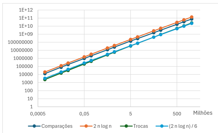
Figura 5: Comparativo entre o número de comparações e trocas e seu compartimento esperado para o melhor caso do quick sort. Escala dílog.
