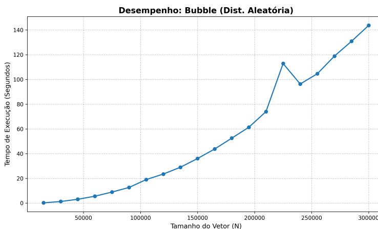
Figura 2: Desempenho Bubble Sort: Caso médio
