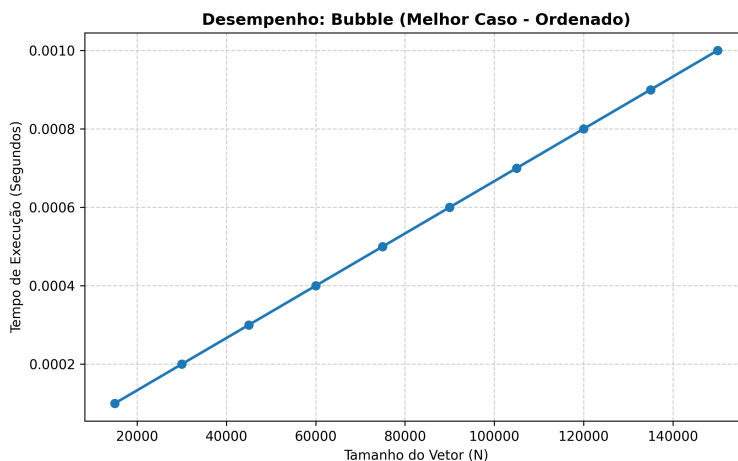
Figura 1: Desempenho Bubble Sort: Melhor caso
