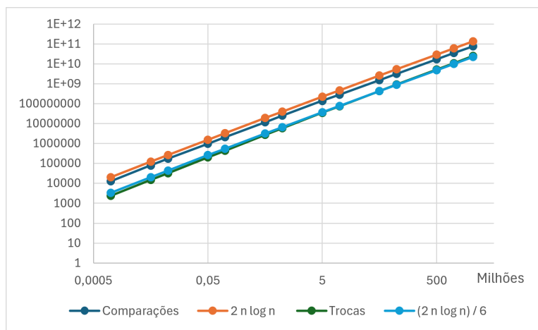
Figura 1: Comparativo entre o número de comparações e trocas e seu comportamento esperado para o melhor caso do quick sort. Escala dílog.
