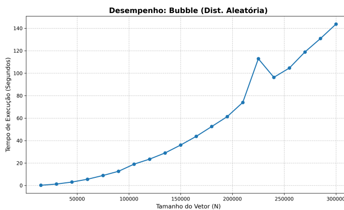
Figura 2: Desempenho Bubble Sort: Caso médio
