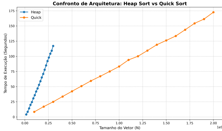
Figura 9: Comparativo de tempo de execução entre Heap Sort e Quick Sort evidenciando a degradação temporal do Heap Sort decorrente de Cache Misses para vetores massivos.
