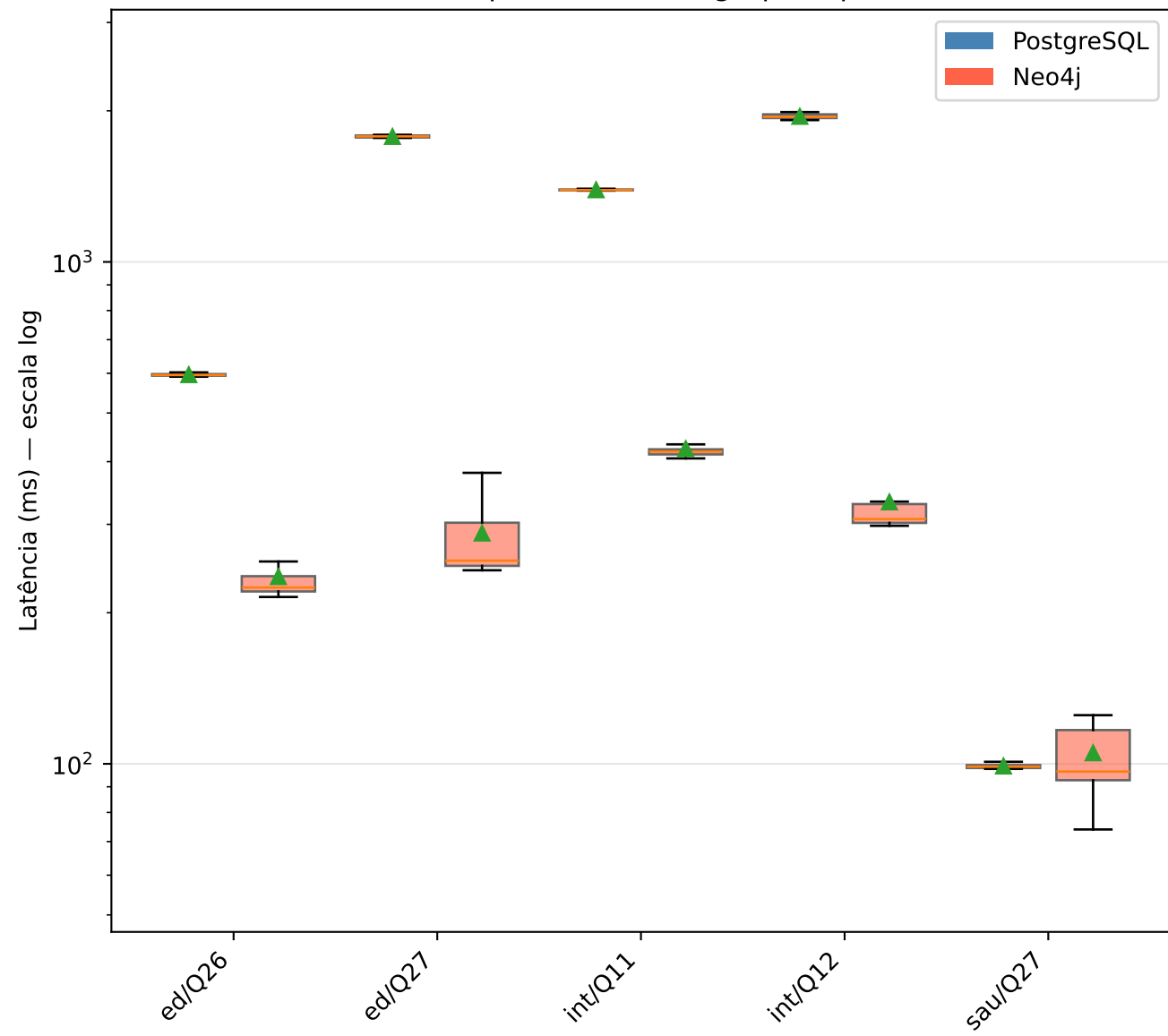
Latência por consulta — grupo Espacial
