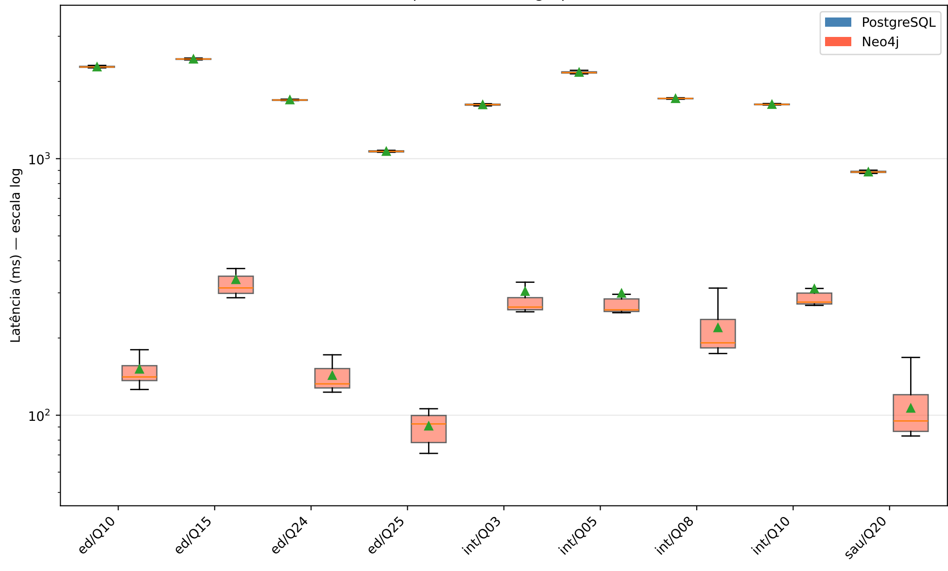
Latência por consulta — grupo Multi-salto
