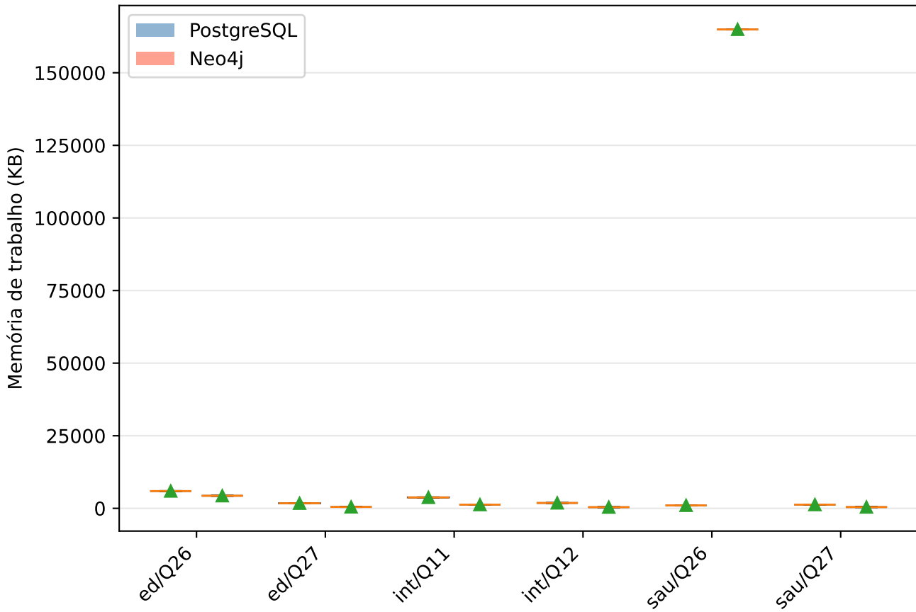
Memória de trabalho por consulta — grupo Espacial
