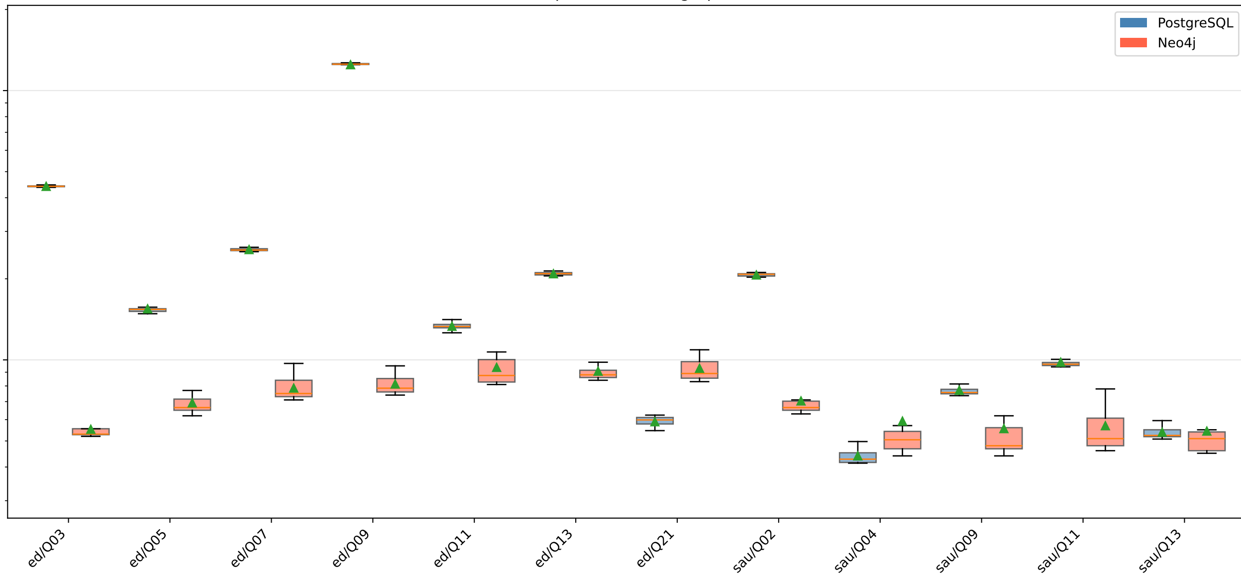
Latência por consulta — grupo Filtro
