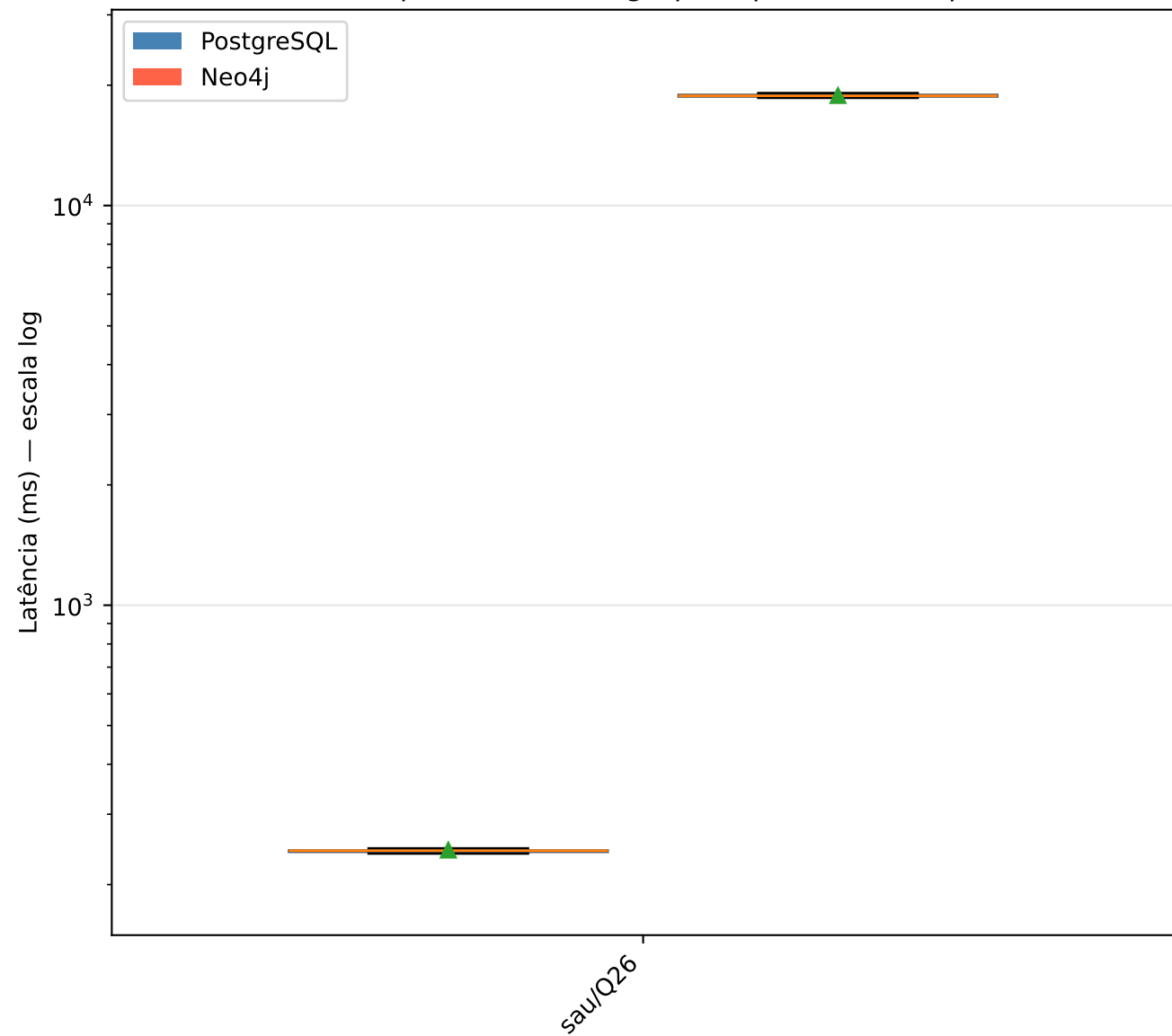
Latência por consulta — grupo Espacial (destaques)
