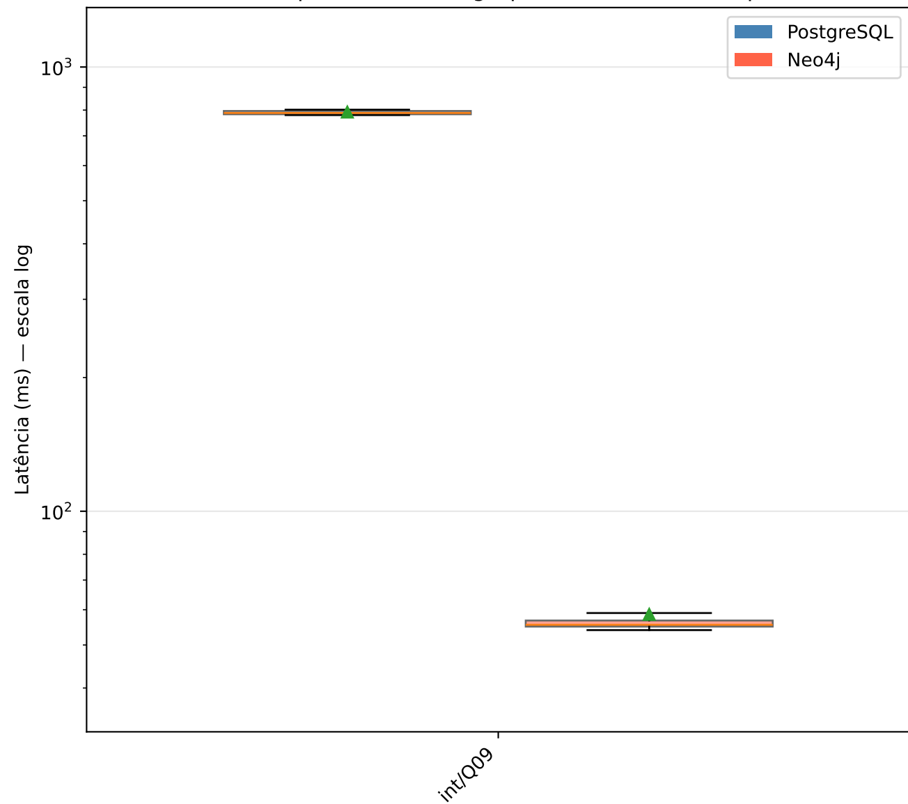
Latência por consulta — grupo Multi-salto (destaques)
