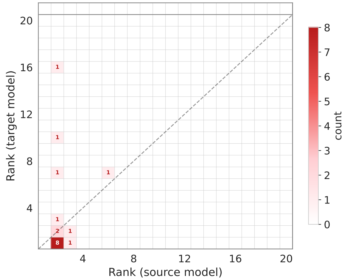
Qwen3-8B → Qwen3-0.6B
