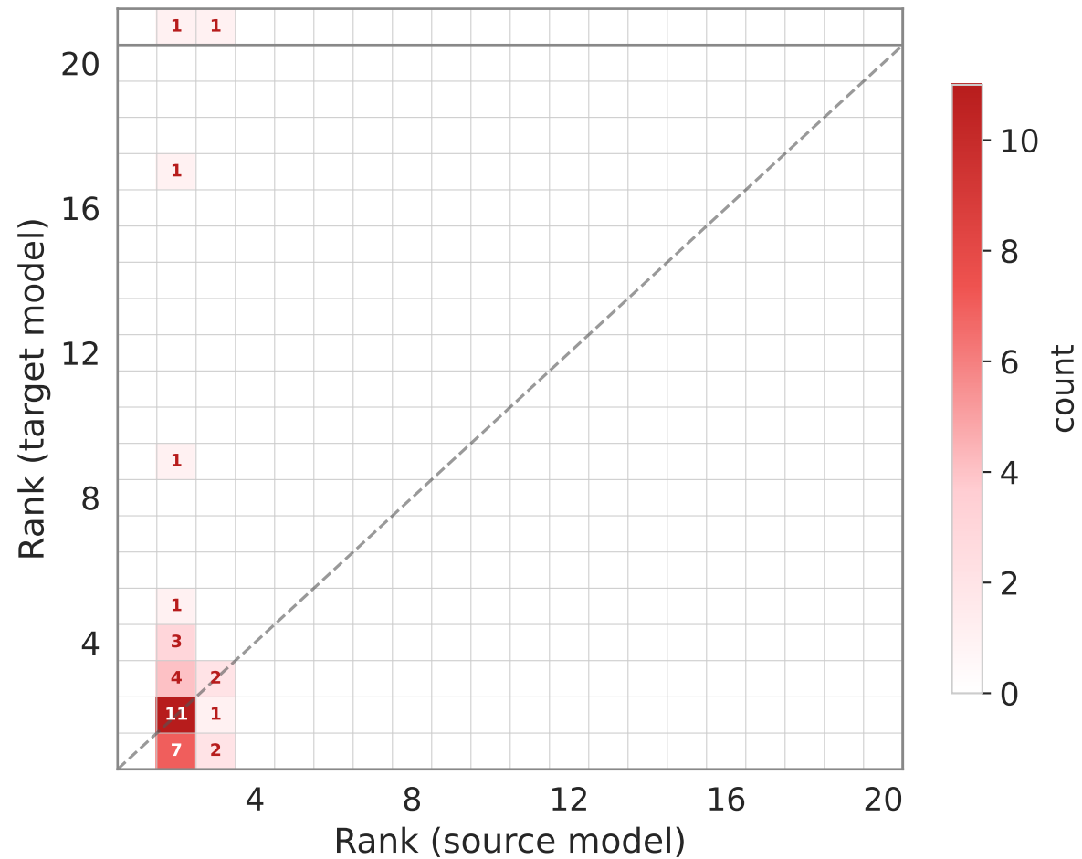
Qwen3-0.6B → Qwen3-8B
