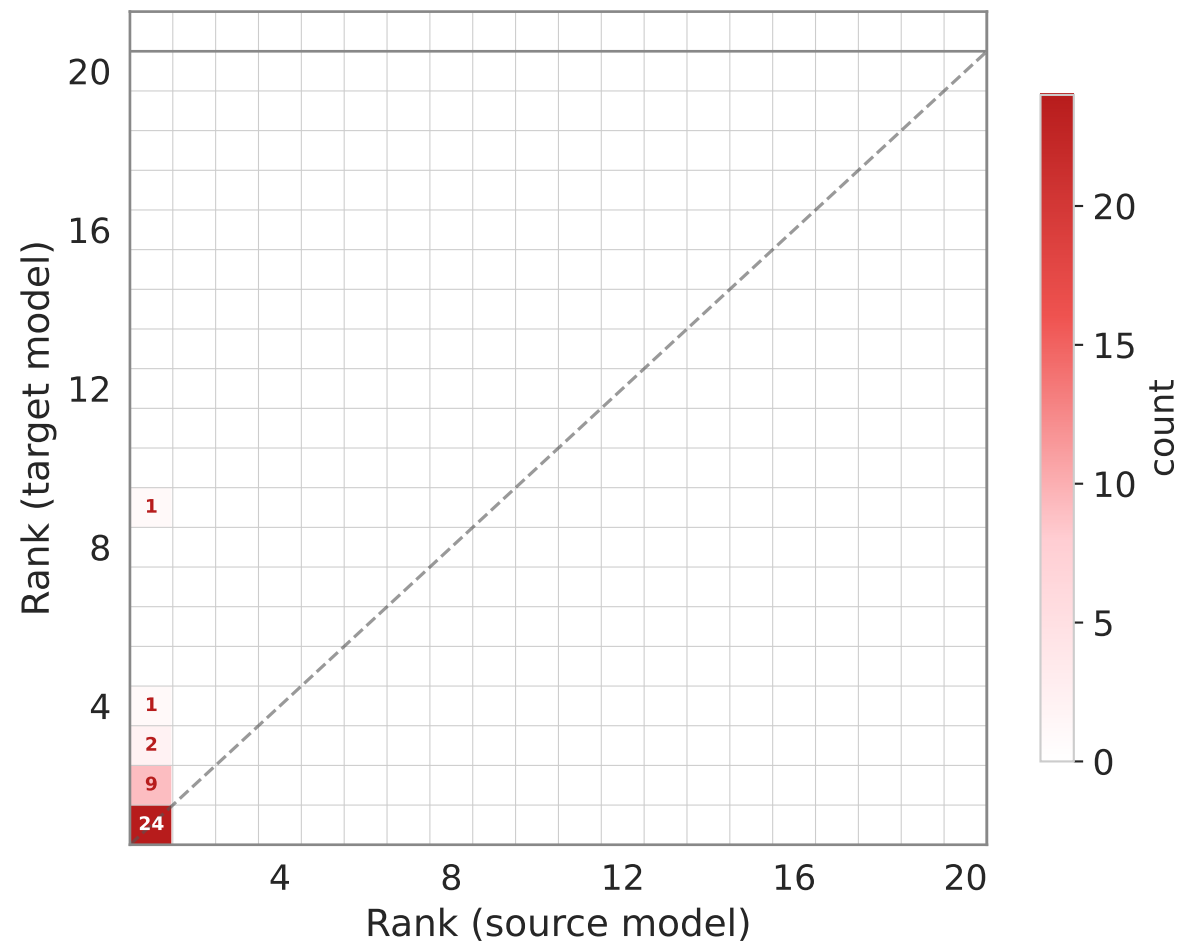
Llama-3.1-8B → Llama-3.2-1B
