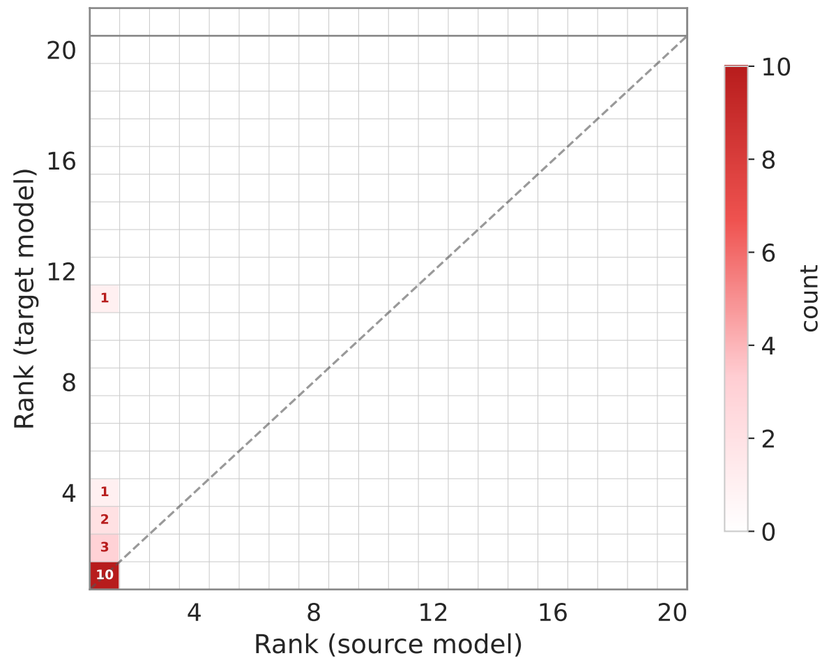
Llama-3.2-1B → Llama-3.1-8B
