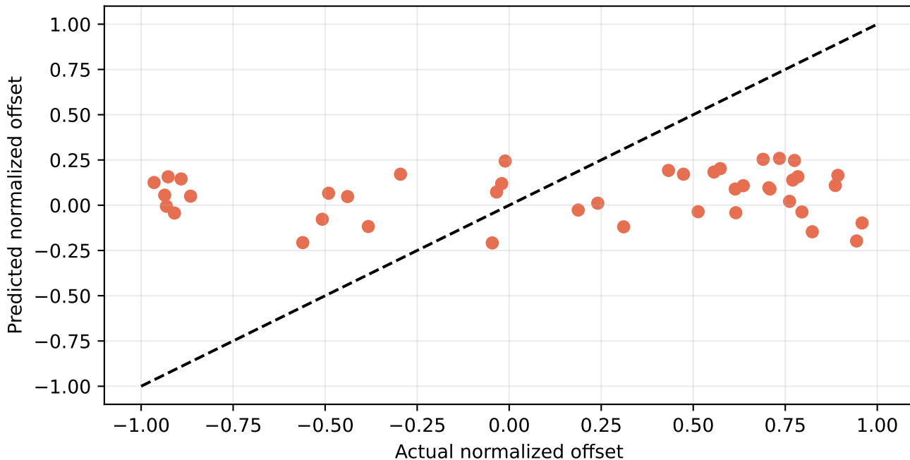
Figure 24. ANFIS actual versus predicted offset
