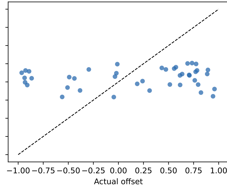
ANFIS
