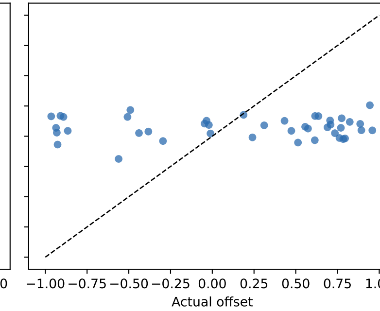
MobileNetV3
