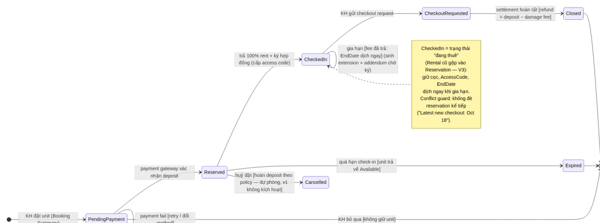
Hình 3: State chart Reservation
