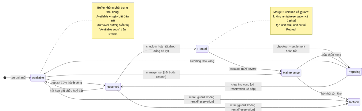
Hình 2: State chart Unit
