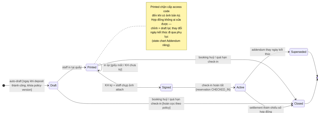
Hình 5: State chart Contract
