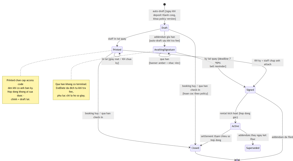
Hình 5: State chart Contract
