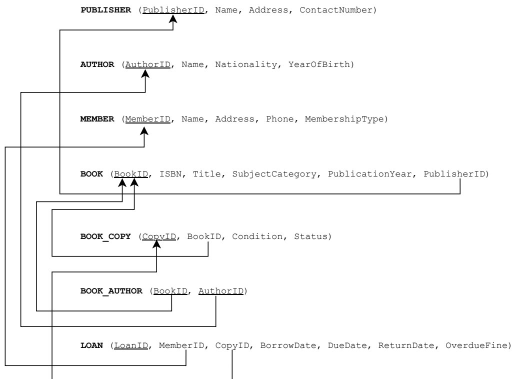
Hình 3: Sơ đồ Mô hình Quan hệ (RDM) từ Báo cáo 2 - Đã xác nhận đạt 1NF, 2NF, 3NF
