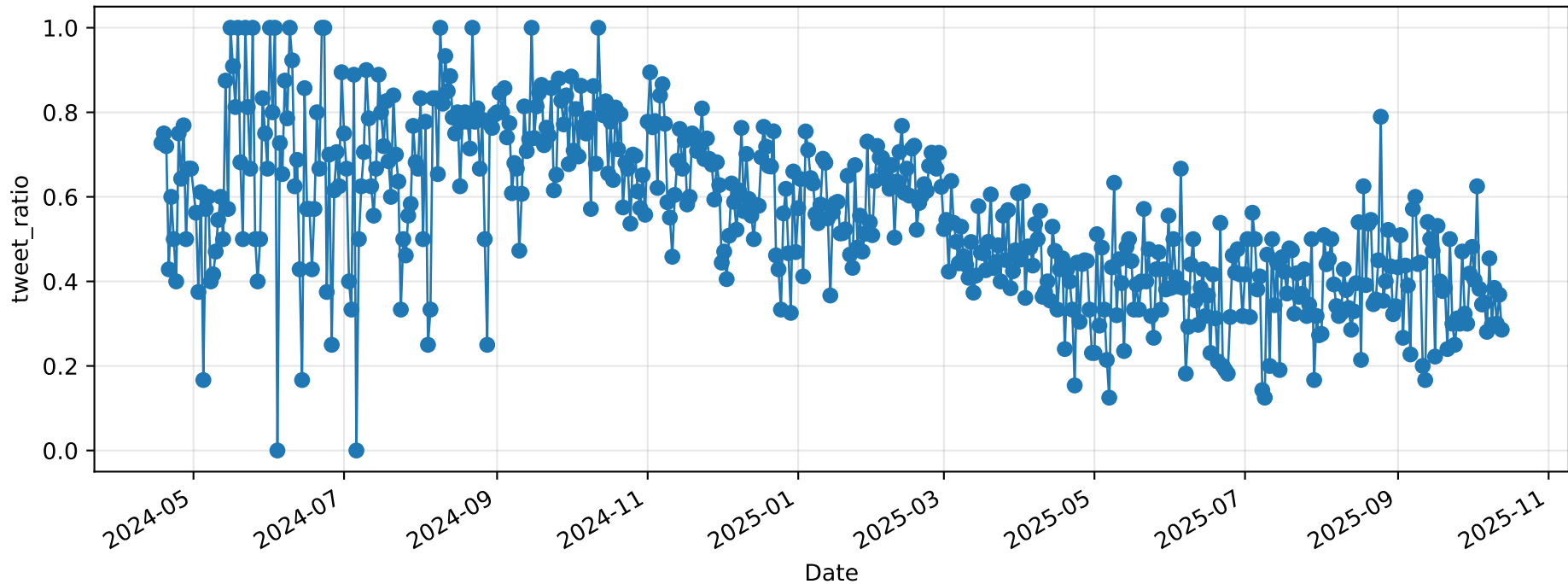
tweet_ratio
