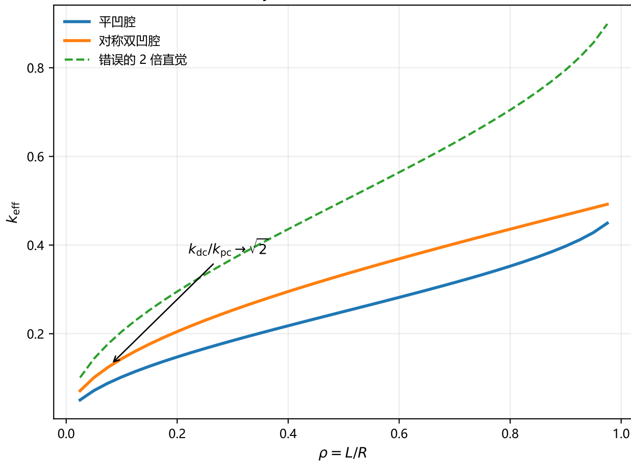
(a) 同一几何比下的有效 Gouy 步长
