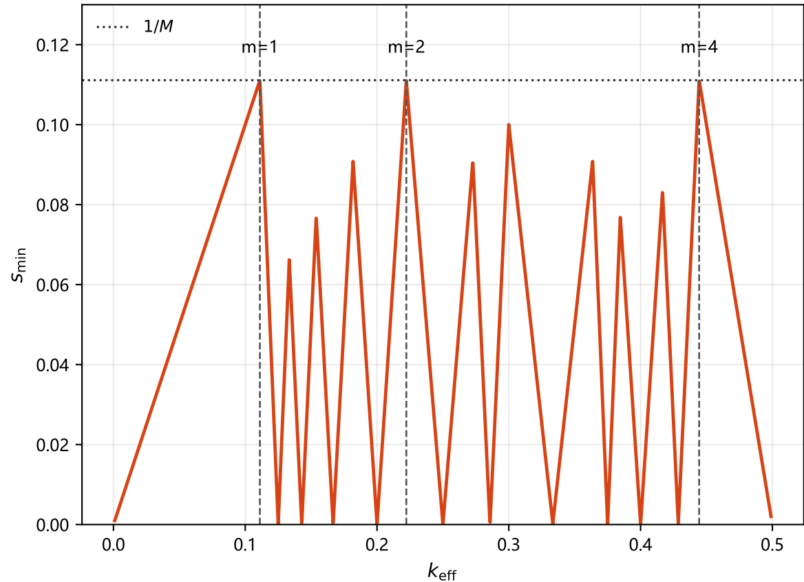
(b) M=9 的解析最优分支
