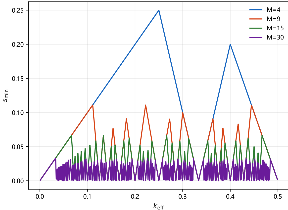
(a) 连续总阶集合的最小间距景观
