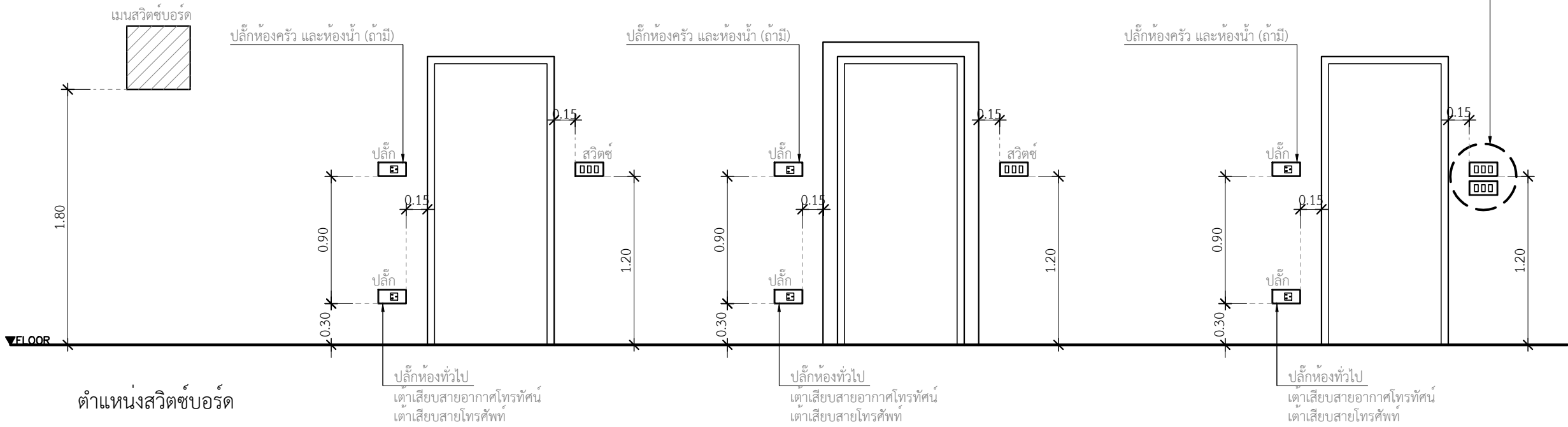
ตำแหน่งสวิตช์และปลั๊กทั่วไป
