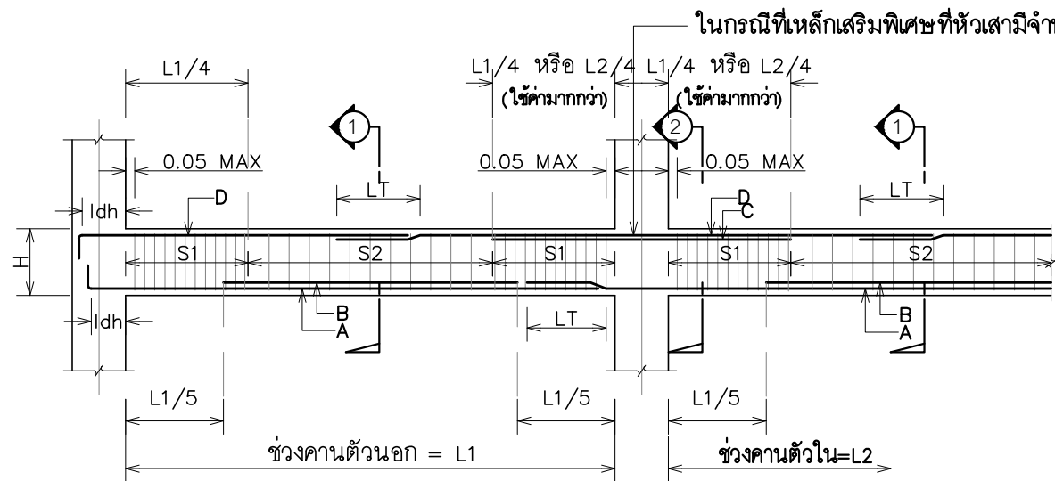
การเสริมเหล็กสำหรับคานต่อเนื่อง TYPE A
