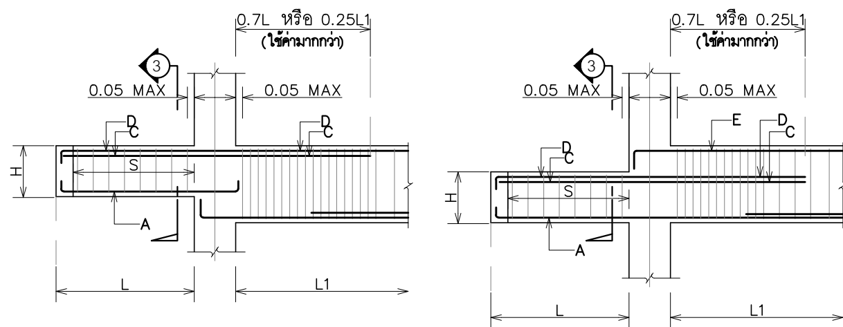
การเสริมเหล็กสำหรับคานยื่น TYPE B
