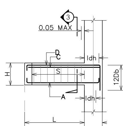
การเสริมเหล็กสำหรับคานต่อเนื่อง TYPE C
