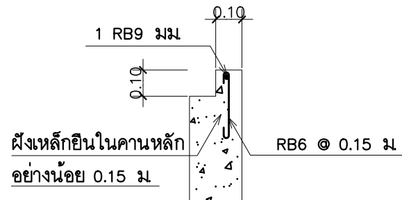
แบบขยายคาน ค.ส.ล. รับพื้นหล่อในที่
