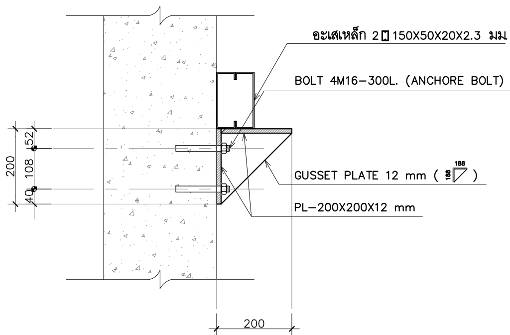
แบบขยายจุดต่อ "J1"
