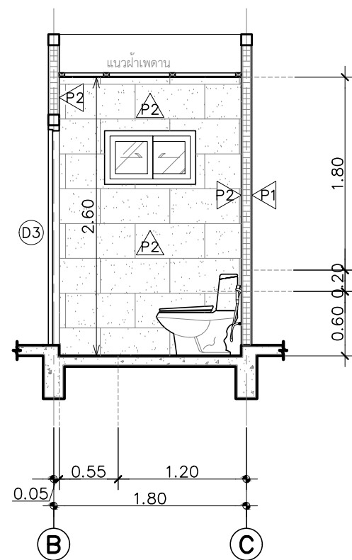
รูปตัด A (ห้องน้ำ WC2) มาตราส่วน 1:50
