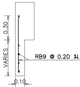
(เสริมใต้คาน)
