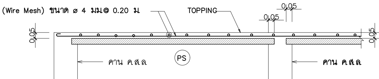
ขยายพื้น TOPPING 1:20
