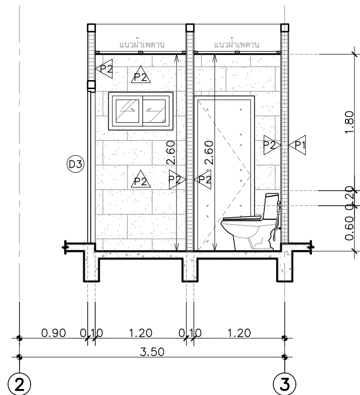
รูปตัด B (ห้องน้ำ WC1, WC2) มาตราส่วน 1:50
