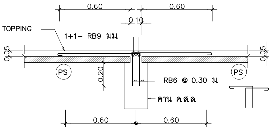
ขยายการวางพื้น (PS) ช่วงภายใน 1:20
