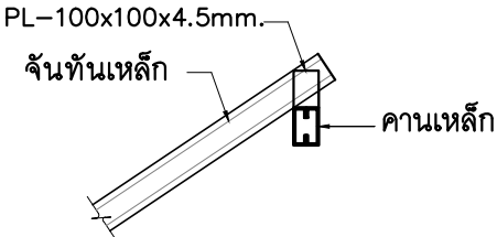
แบบขยาย : การยึดจันทันกับคานเหล็ก
