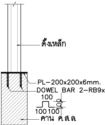
แบบขยาย : การยึดดั่งเหล็กกับคาน ค.ส.ล.
