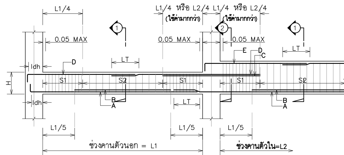
การเสริมเหล็กสำหรับคานต่อเนื่อง TYPE C
