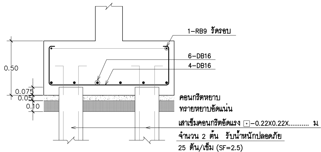
แบบขยายฐานราก F2 SCALE 1: 20
