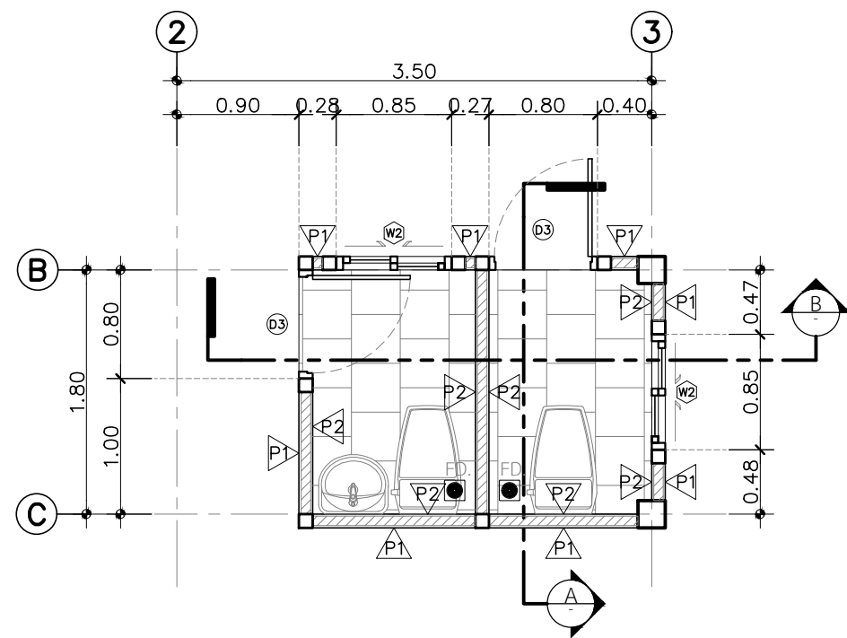
แปลน ห้องน้ำ WC1, WC2 มาตราส่วน 1:50
