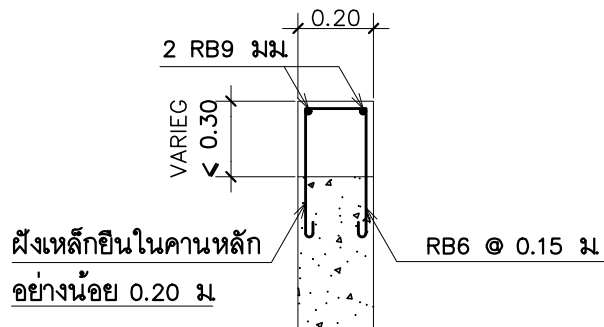
แบบขยายคาน ค.ส.ล. รับพื้นหล่อในที่
