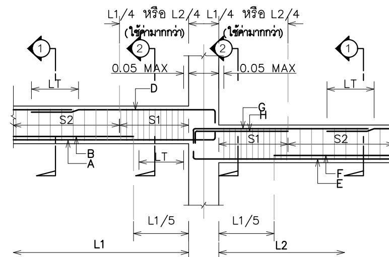
การเสริมเหล็กสำหรับคานต่างระดับ
