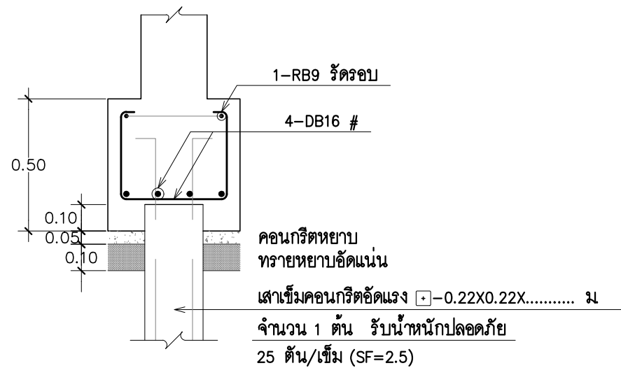
แบบขยายฐานราก F1 SCALE 1: 20
