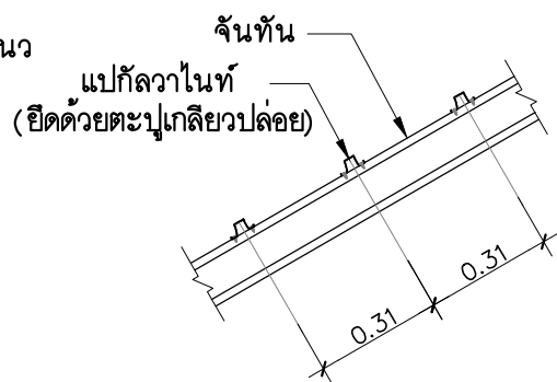
แบบขยาย : การติดตั้งแป็กฉวไนท์
