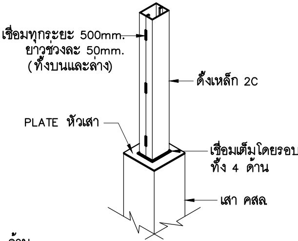
แบบขยาย : การวางดั่งบนเสา คสล.
