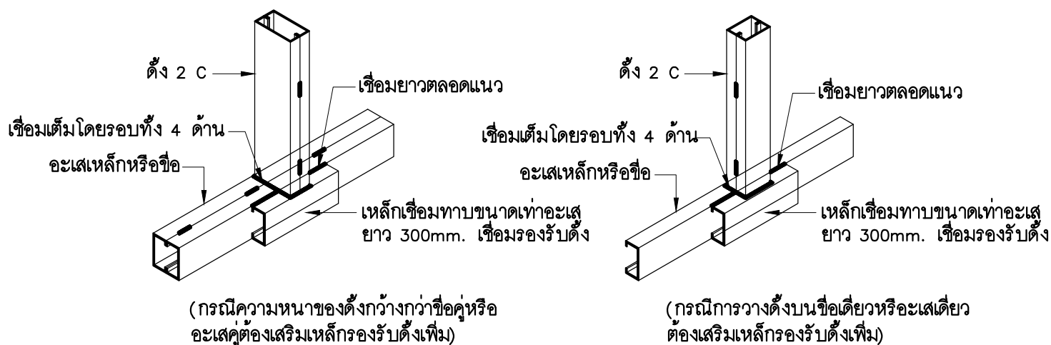
แบบขยาย : การวางดิ่งบนอะเส
