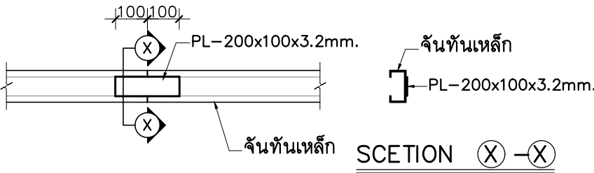
แบบขยาย : การต่อเหล็กจันทัน
