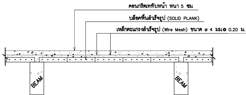
แบบขยายรูปตัดพื้นสำเร็จ (SOLID PLANK) รูปตามขวาง
