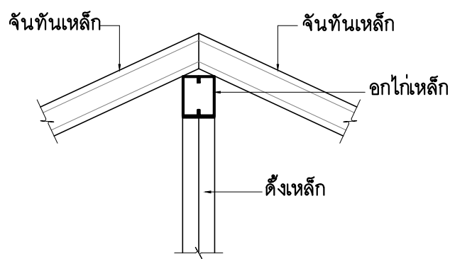
แบบขยาย : การยึดจันทันเหล็กกับอกไก่เหล็ก
