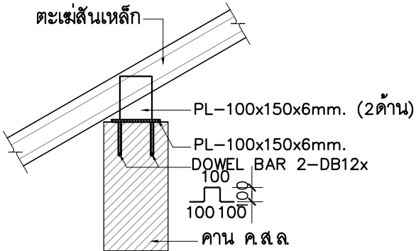
แบบขยาย : การยึดตะแคงเหล็กกับคาน ค.ส.ล.
