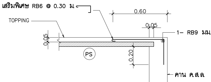
ขยายการวางพื้น (PS) บริเวณคานริม 1:20
