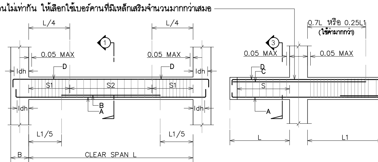
การเสริมเหล็กสำหรับคานช่วงเดียว
