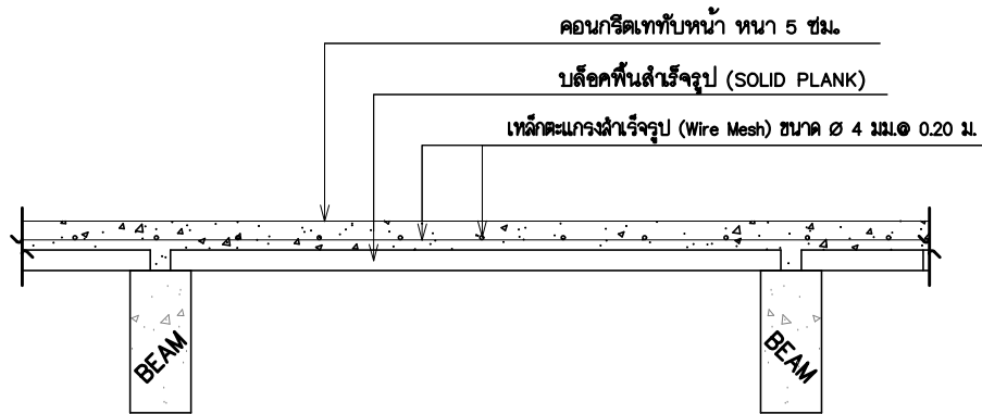
แบบขยายรูปตัดพื้นสำเร็จ (SOLID PLANK) รูปตามยาว
