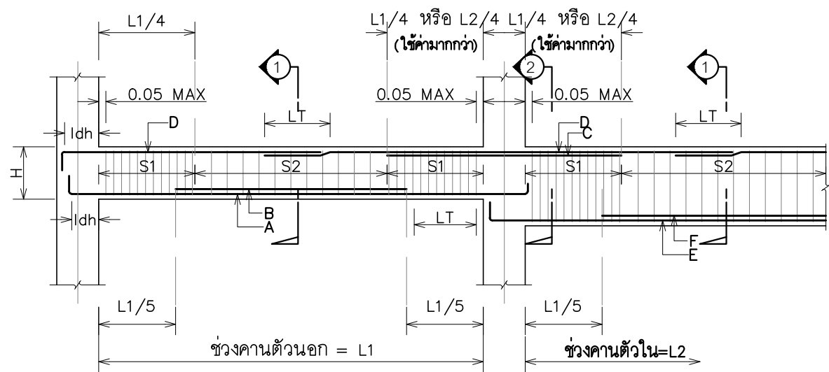
การเสริมเหล็กสำหรับคานต่อเนื่อง TYPE B
