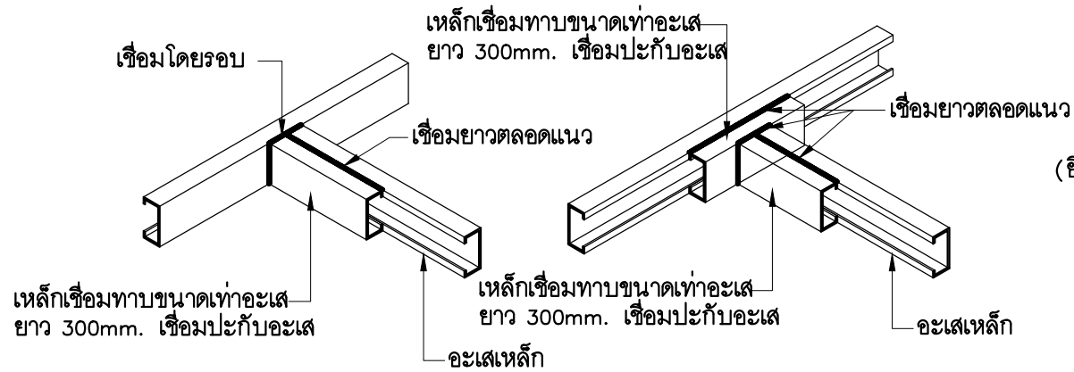
แบบขยาย : การเชื่อมชนอะเสเหล็ก
