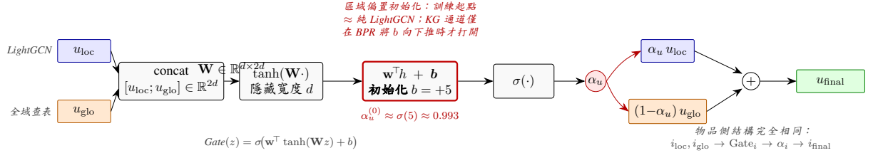
Figure 4: 區域偏置融合閘，以使用者側為例。區域表示 u_{loc} （來自 LightGCN）與全域表示 u_{glo} （直接查全域使用者表）先串接，經一小型 MLP（隱藏寬度 d 、 \tanh ），標量 logit 再加上 初始化偏置 b = +5 後送入 sigmoid（式 (3.24)）。所得 \alpha_u \in (0, 1) 構成凸組合 u_{final} = \alpha_u u_{loc} + (1 - \alpha_u) u_{glo} 。偏置初始化使 \alpha_u^{(0)} \approx 0.993 ，訓練起點實質上等同純 LightGCN；KG 通道僅在 BPR 梯度將 b 向下推時才打開（第 3.8.3 節）。物品側結構完全相同：另一個架構一致的 Gate_i 將 (i_{loc}, i_{glo}) 映射至 \alpha_i 與 i_{final} ，其偏置亦初始化為 +5 。
