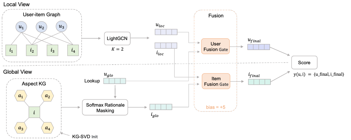
Figure 1: RA-GARK 架構。
