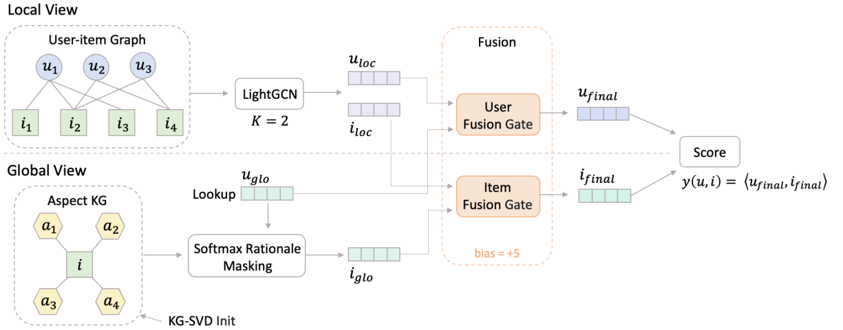
Figure 1: RA-GARK 架構。
