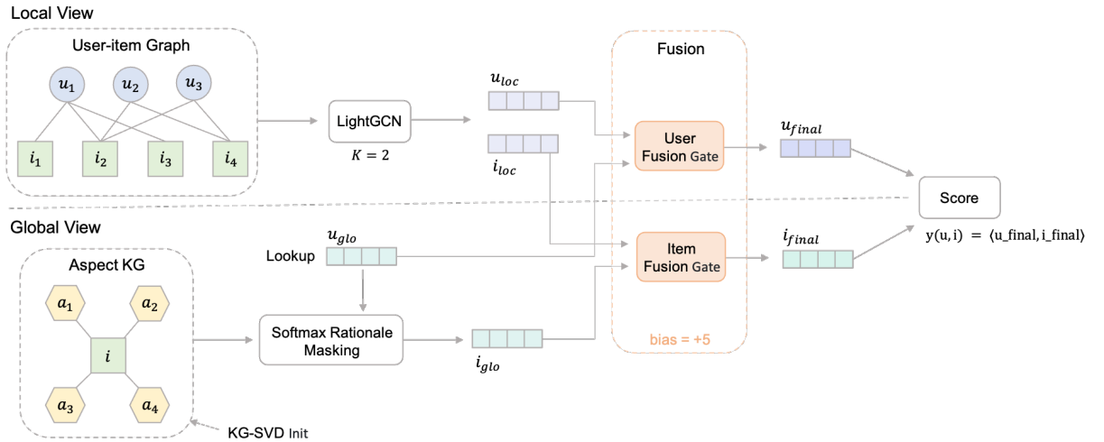
Figure 1: RA-GARK 架構。
