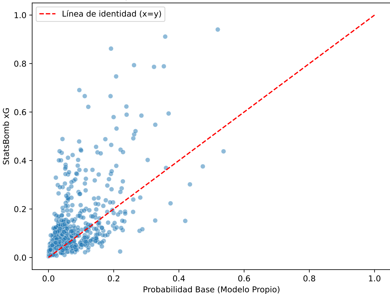
Comparación: Modelo Base vs StatsBomb xG
