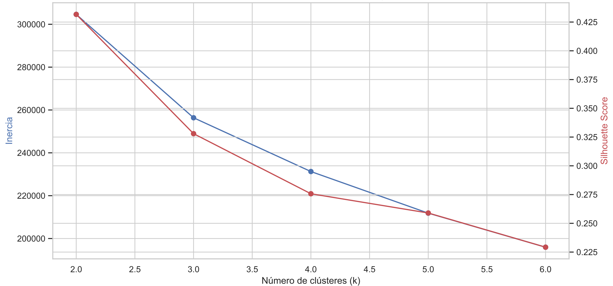
Evaluación de K-Means: Método del Codo y Silueta
