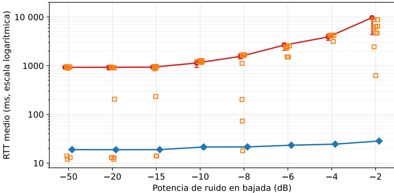
RTT medio
