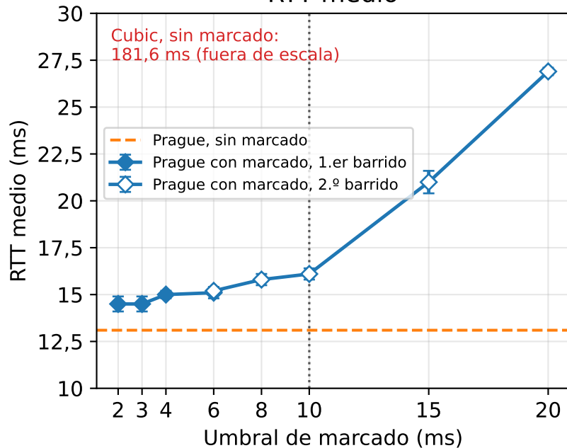
RTT medio
