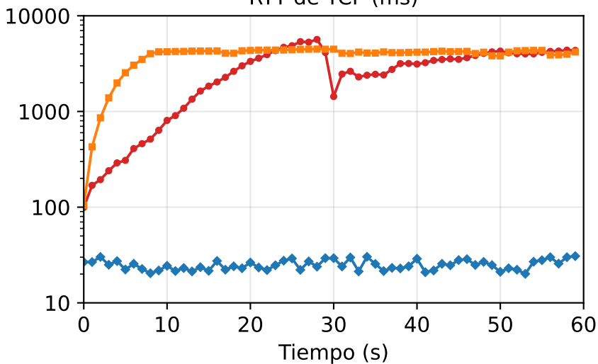
RTT de TCP (ms)
